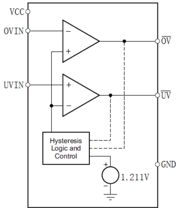
图 4 原理框图
